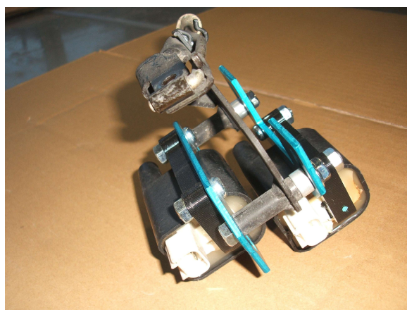
図2、SP2 コイル取付(フロントから見た場合) 6 * 50mmボルト、6 * 6mmスペーサ使用。
