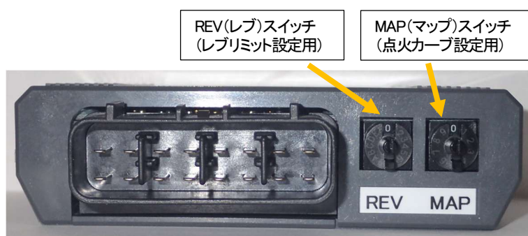
SP2 コントロールユニット
