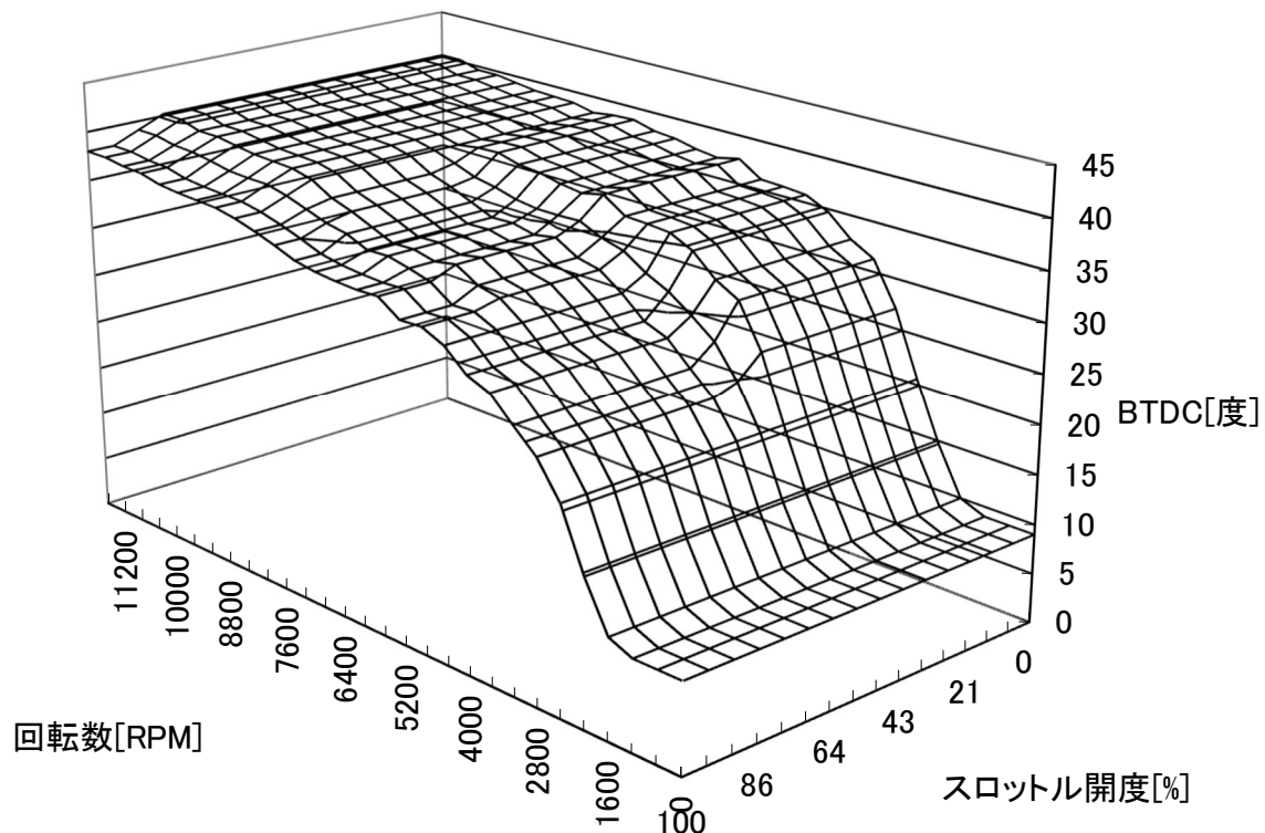
SP2点火マップ(0マップ) H.CBR1100XX
