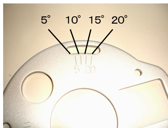
図4、取付ボルトの中心が10° のマーク に一致するように装着する
