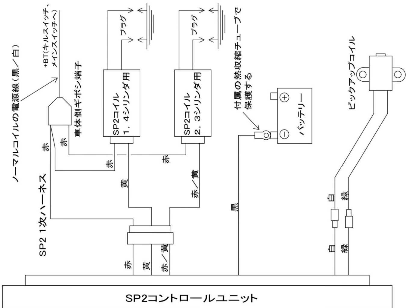
図7、SP2点火システム配線図
