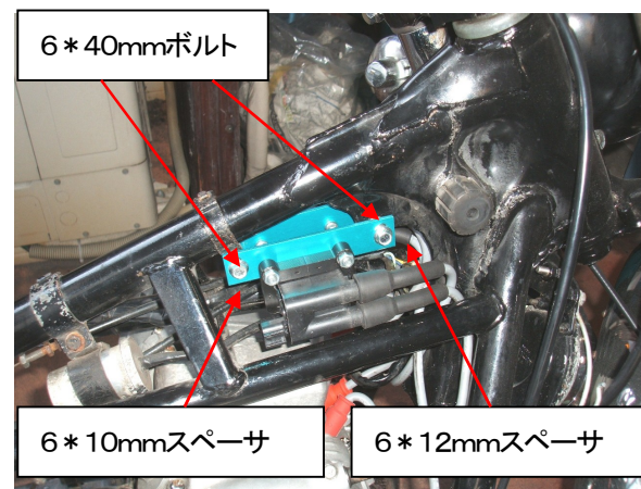
図6、SP2 コイルの装着
