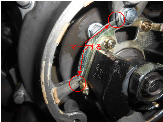
図1 カバー取外し、合いマーク
