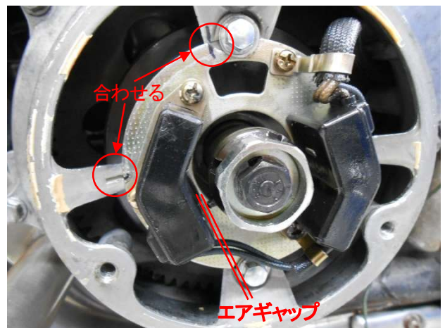
図4 パルスジェネレーターの取付位置、エアギャップの確認調整
