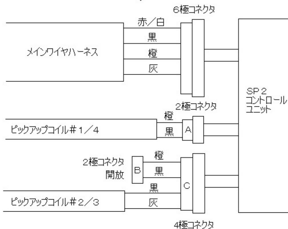
SP 2 コントロールユニット 接続図
