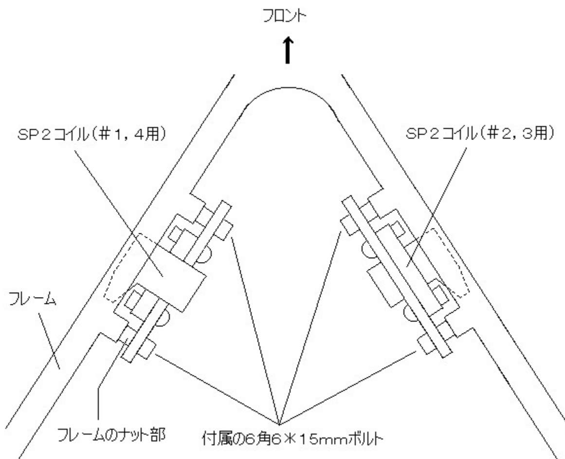
SP2 コイル装着図(上から見た図)
