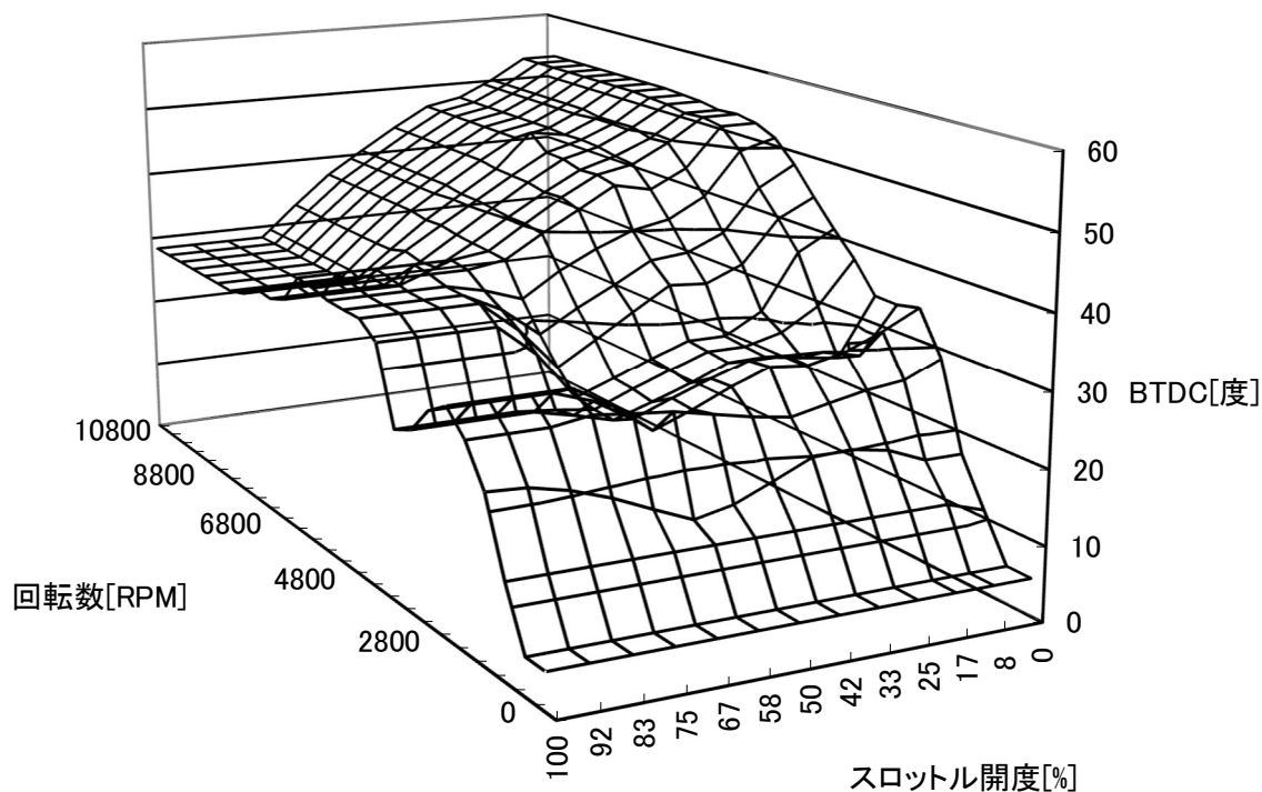
SP2点火マップ(0マップ) Y.XJR1300-2
