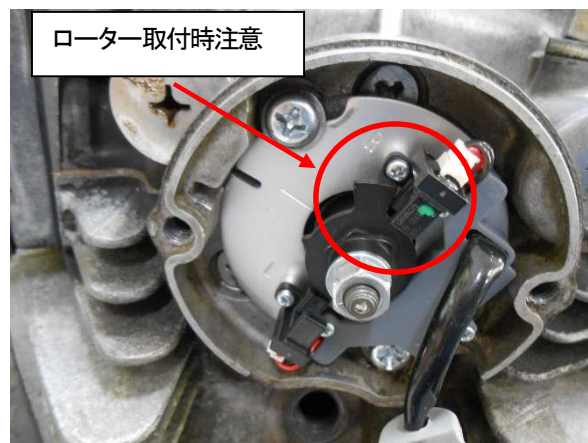
図4、タイミングプレートの仮止め及び タイミングロータ取付
