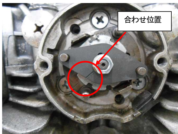
図3、ガバナストッパーの取付
