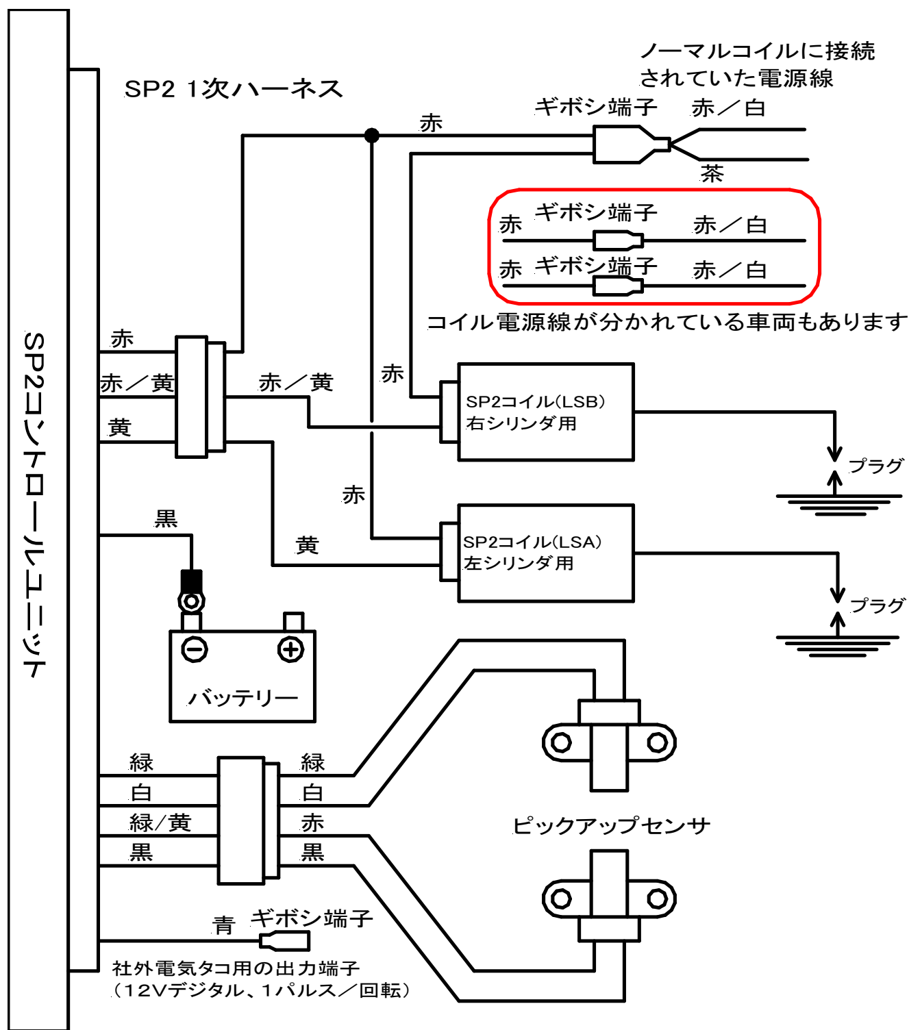
図9、SP2点火システム配線図
