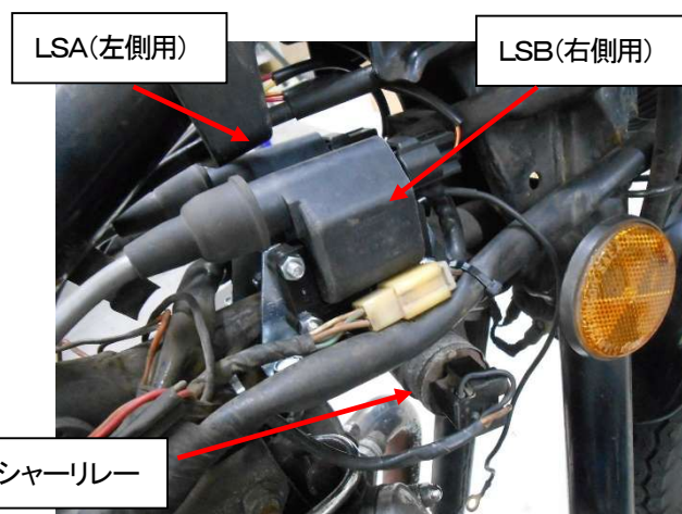
図8、SP2 コイルの装着
