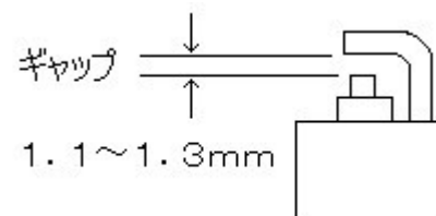
図6、フレームの下に回し固定する
