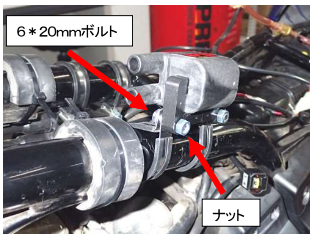
図5、フレームの上で仮組みする
