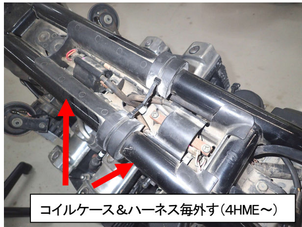
図2、ノーマルコイルの取り外し(4HME～4HML)
