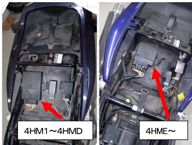
図3、イグナイタの取り外し(4HM1～4HMD)
