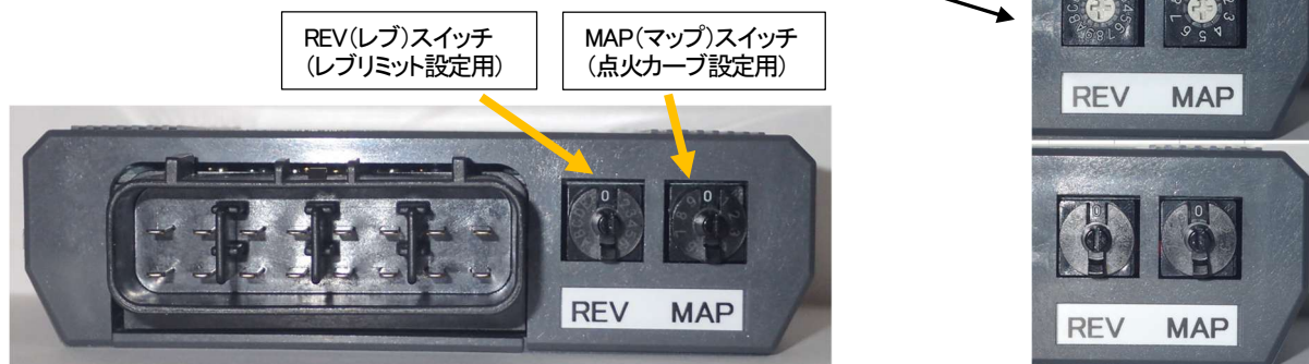
SP2 コントロールユニット
