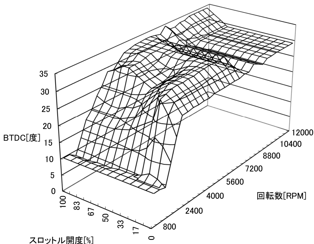
SP2点火マップ(0マップ) K.ZRX1100
