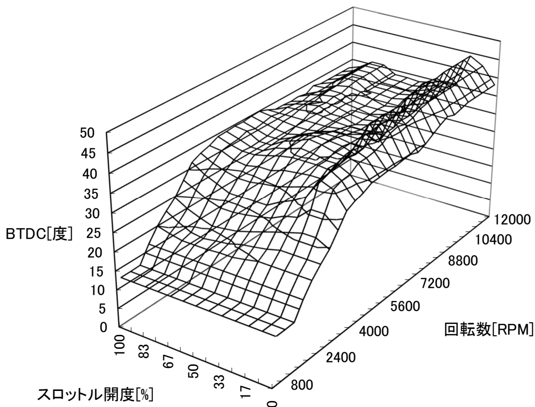
SP2点火マップ(0マップ) K.ZEPHYR750-2
