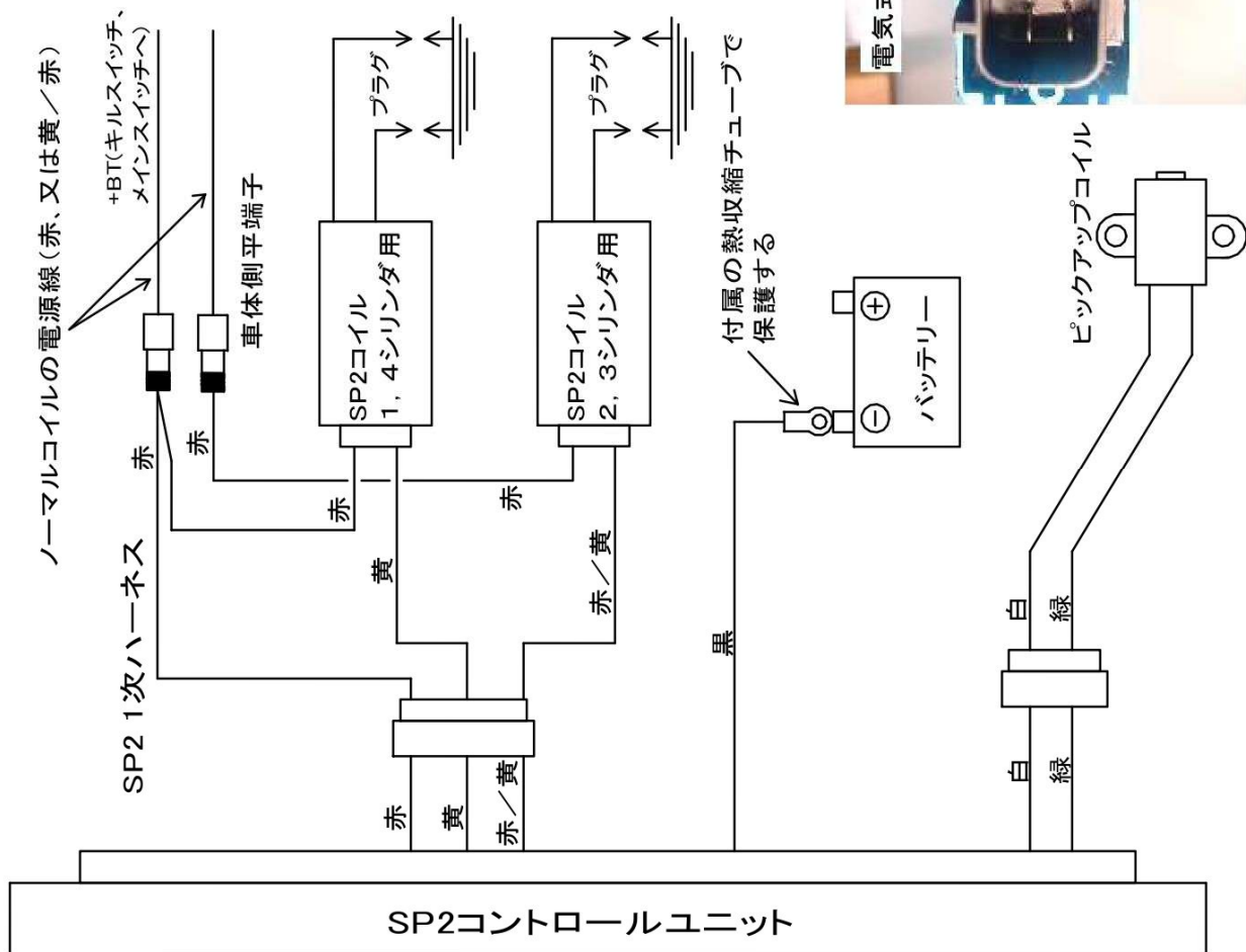
図7、SP2点火システム配線図
