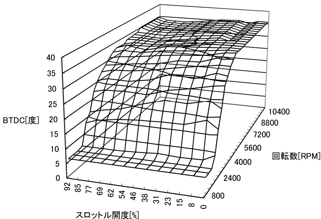
SP2点火マップ(0マップ) S.DR-Z400S
