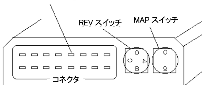
社外品タコメータ用信号出力線(12V1パルス／回転)
