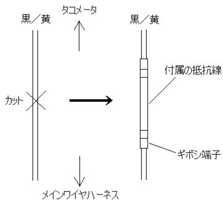
タコメータ下部、抵抗挿入位置
