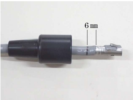
3、コネクタ金具圧着部から6mmのところにマジック等で印をつける。
