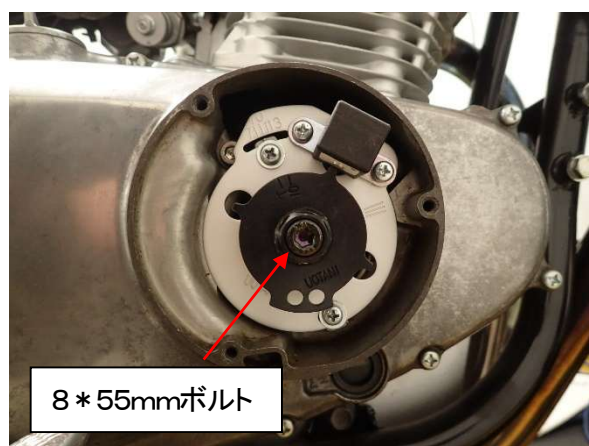
図4、タイミングロータの取付
