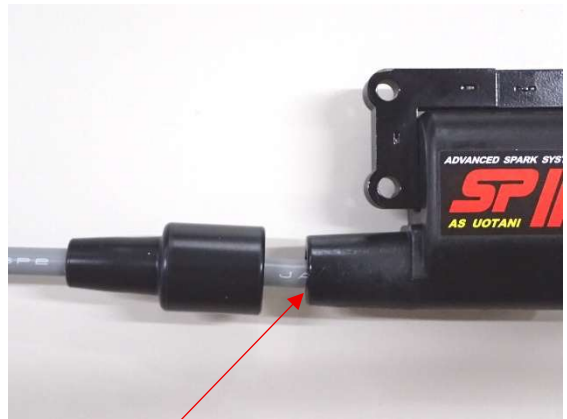
4、6mmの印まで (コイル穴底部まで) コイルに押し込む。
