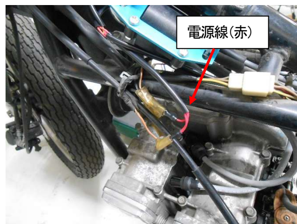
図6、電源線の接続
