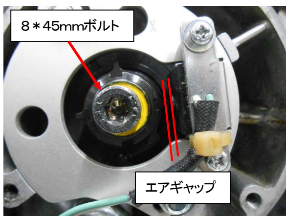
図3、タイミングロータの取付てエアギャップを0, 4~0, 6mmに合わせる
