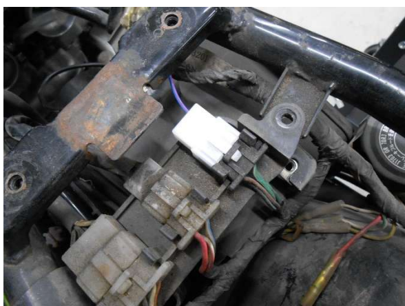
図5、オイルプレッシャースイッチ接続コネクタの装着
