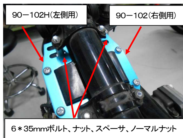
図4、SP2コイルの装着
