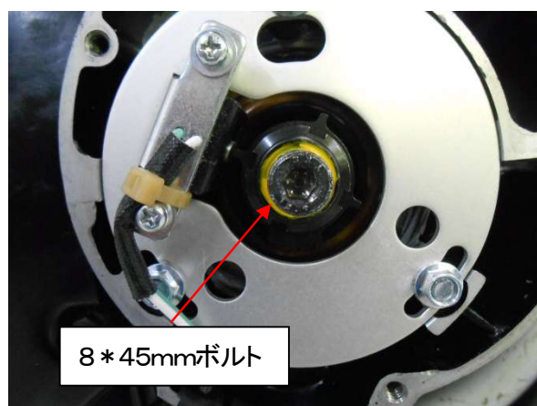
図3、タイミングローターの取付
