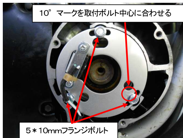
図2、SP2 タイミングプレート(ピックアップコイル)の取り付け
