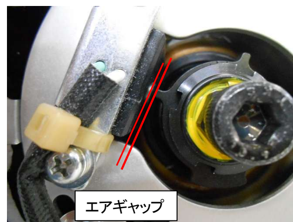
図4、エアギャップを0.4~0.6mmに合わせる
