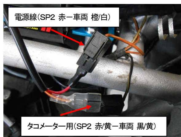
図6、タコメーター用端子は使用しない場合ショートに注意すること
