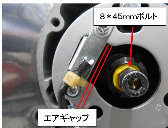
図3、タイミングローターの取付 エアギャップを0, 4~0. 6mm に合わせる
