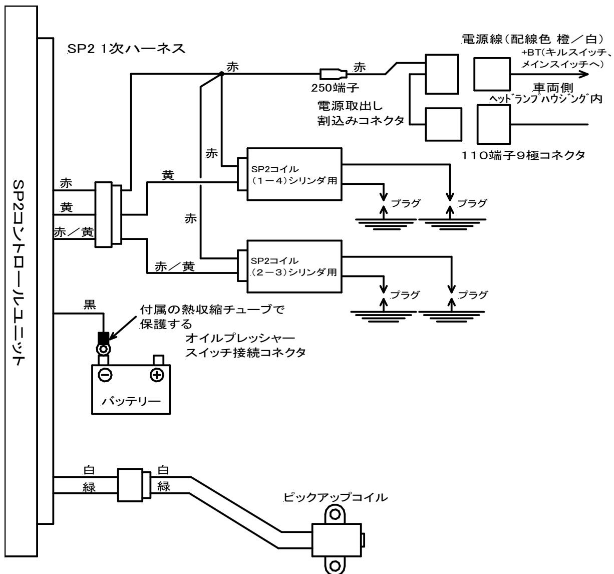
図7、SP2点火システム配線図
