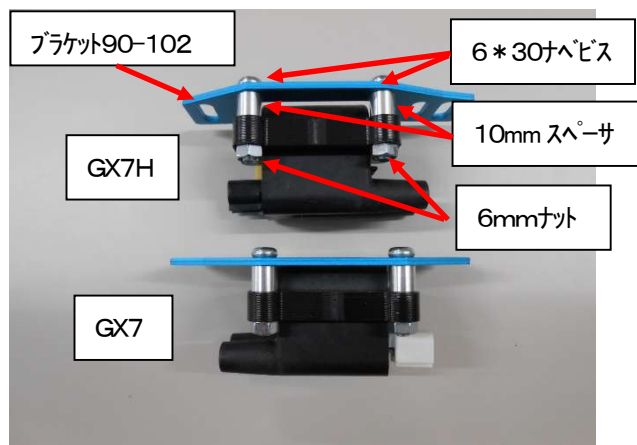
図4、コイル組立図 (キットのコイルは組立済)
