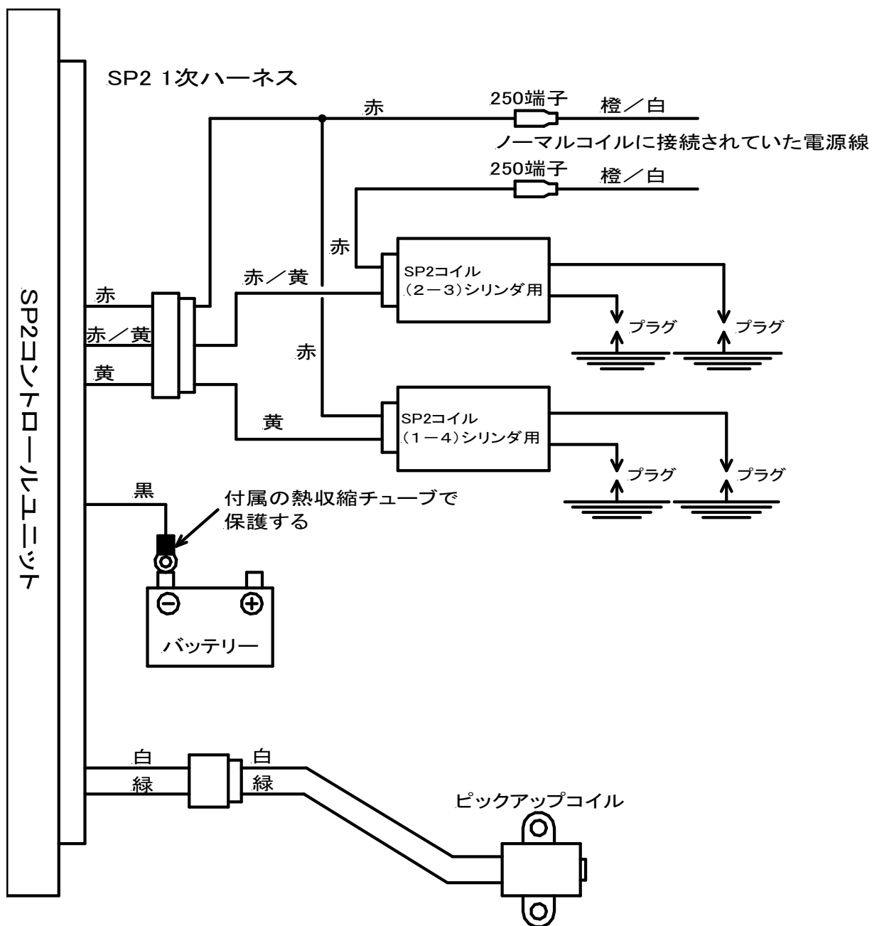
図7、SP2点火システム配線図
