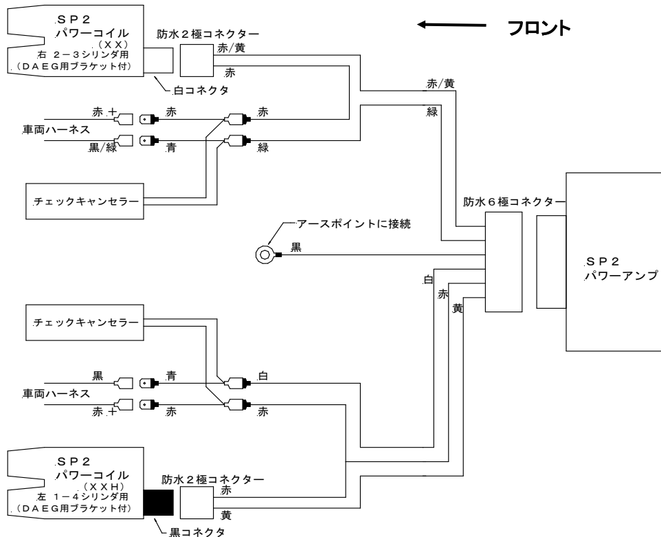
図1 配線図
