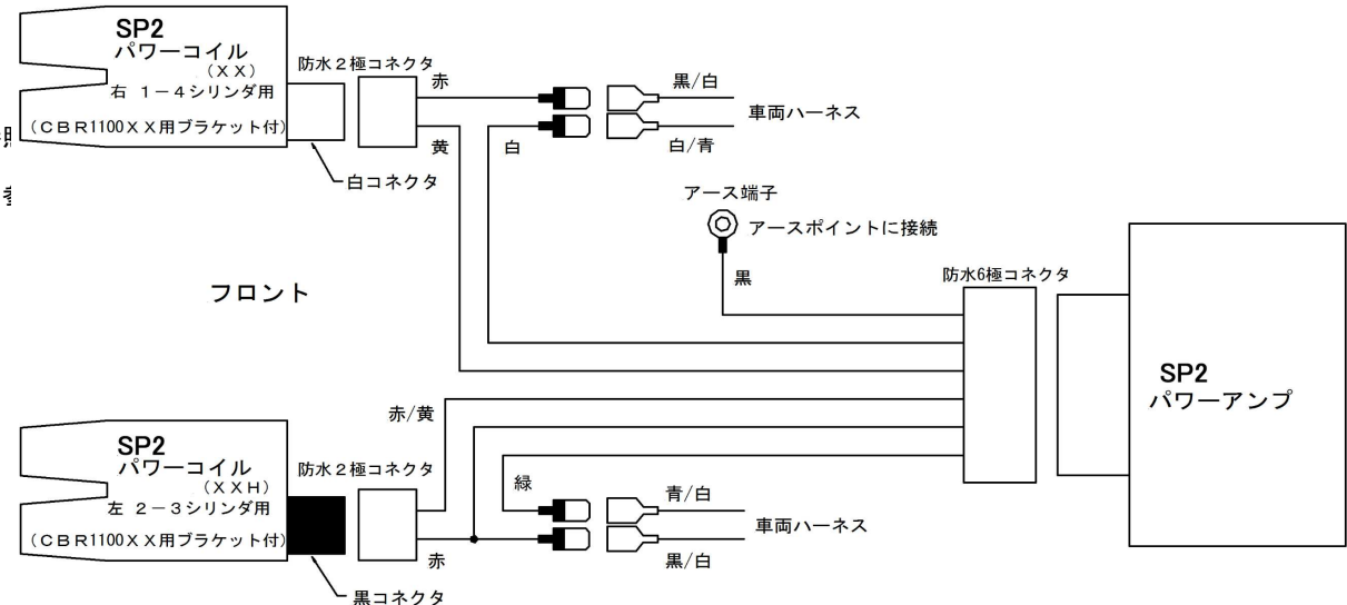
図2 配線図
