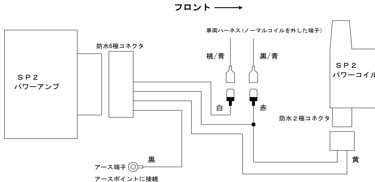
図1配線図
