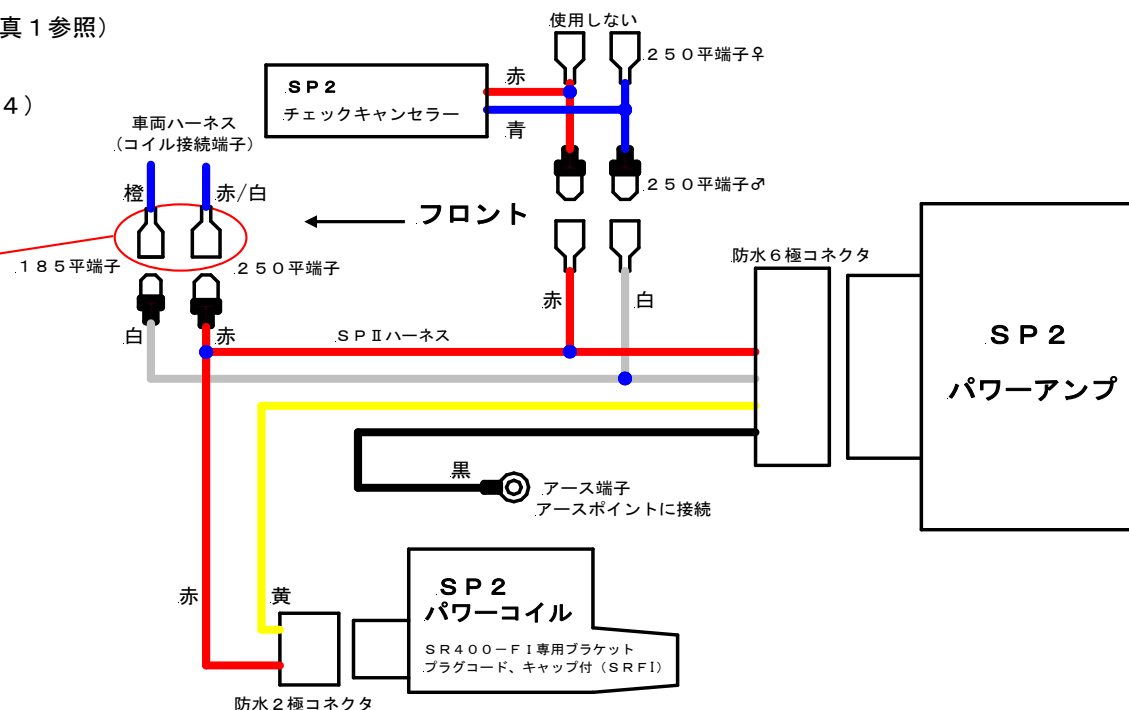
図1配線図
