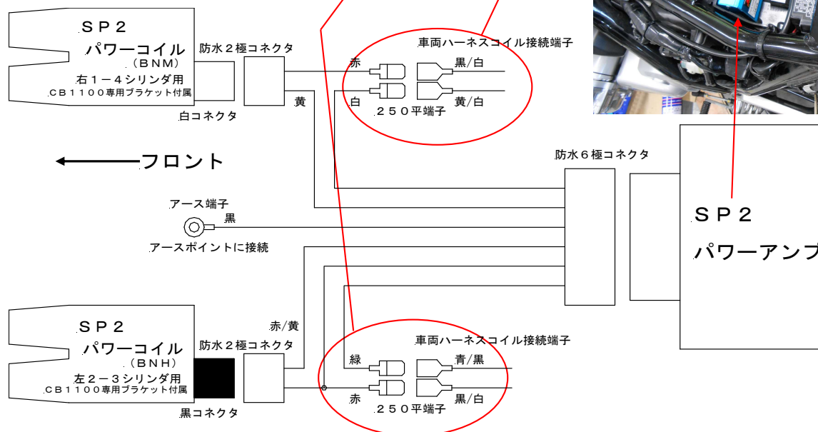
図2配線図
