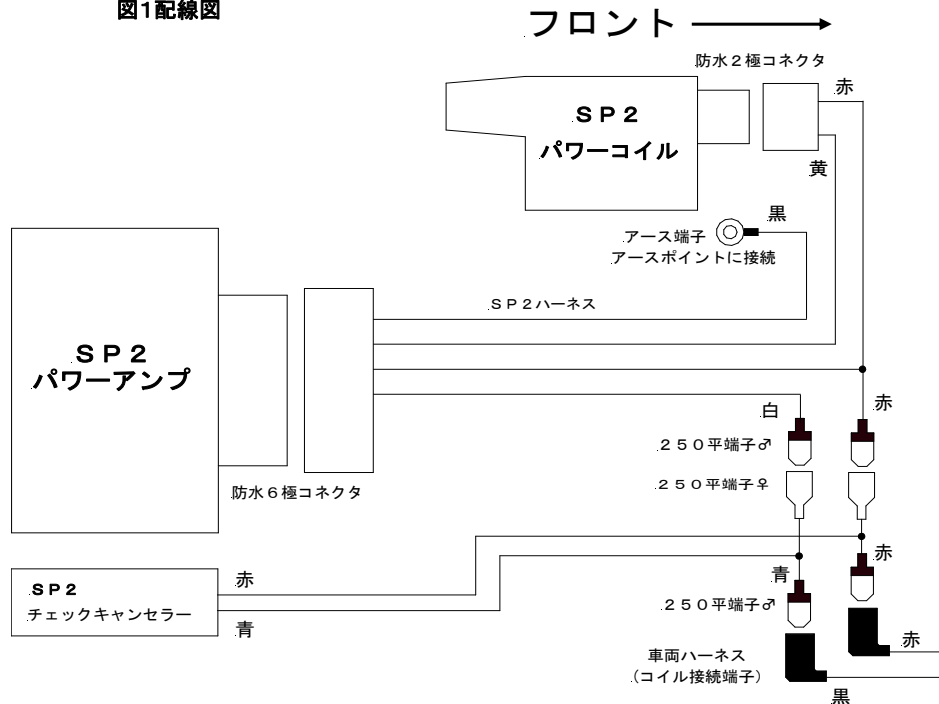
図1配線図
