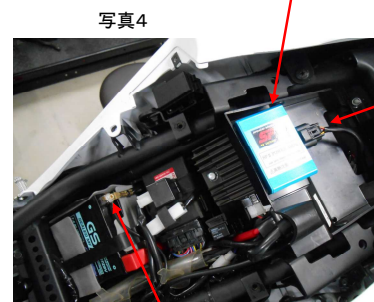
写真4 アース端子バッテリーマイナス端子に接続
