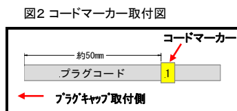
図2 コードマーカー取付図
