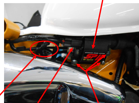
防水2極コネクタ
