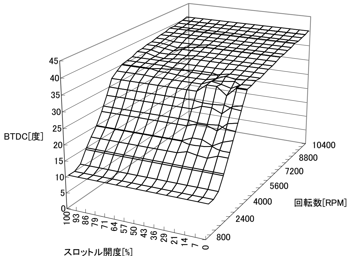
SP II 点火マップ(0マップ) H.CB750
