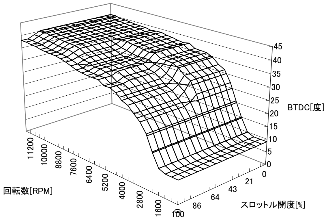
SP II 点火マップ(0マップ) H.CBR1100XX
