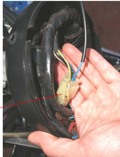
カブラの黄/緑端子を引き抜き その後にSP II 端子(青)を差し込む
