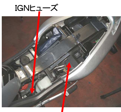
図1、ノーマルイグナイタ
