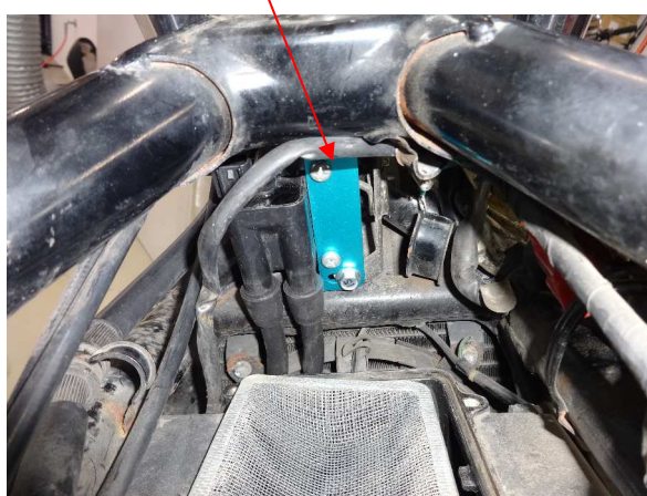
図6、図7、SP II イグニッションコイルの取付け
