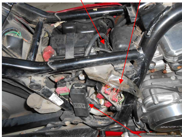
図2、ノーマルイグナイタを外す ヒューズ交換
