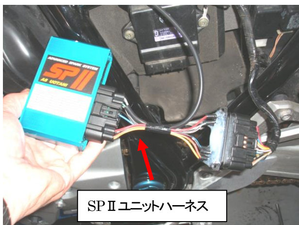
図1、SP II コントロールユニットの接続
