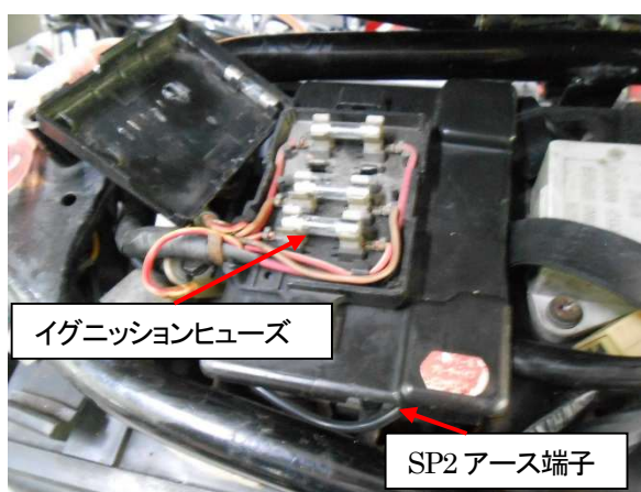
図6、ヒューズの交換
