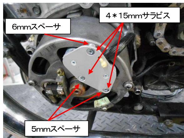
図2、SP2 タイミングプレート(ピックアップコイル)の装着
