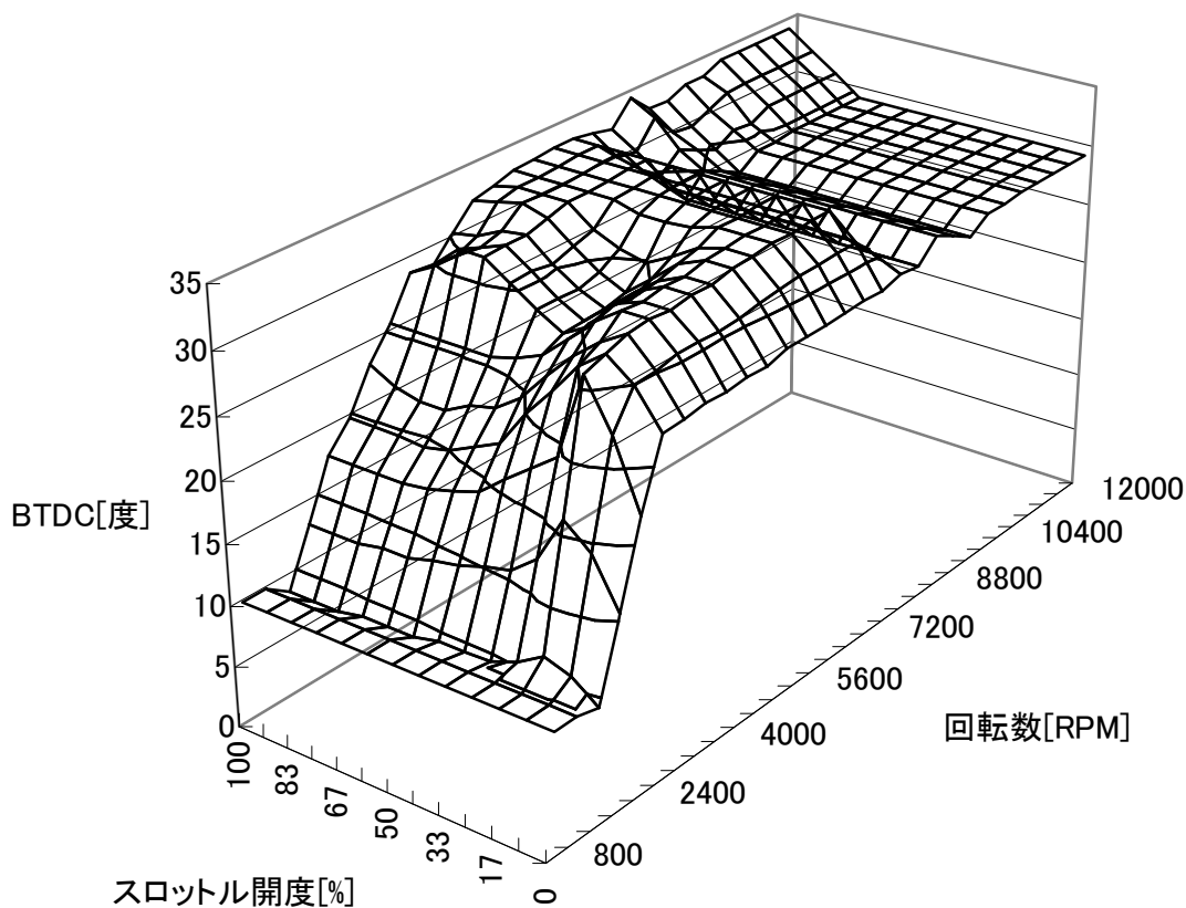
SP II 点火マップ(0マップ) K.ZRX1100
