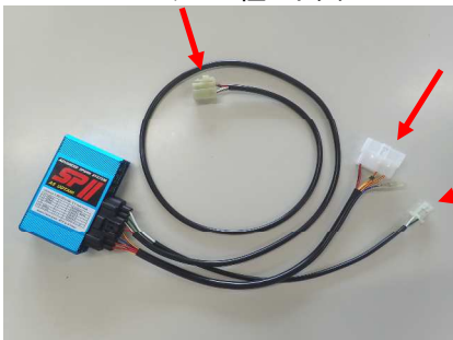
図4、ユニットハーネスの接続
