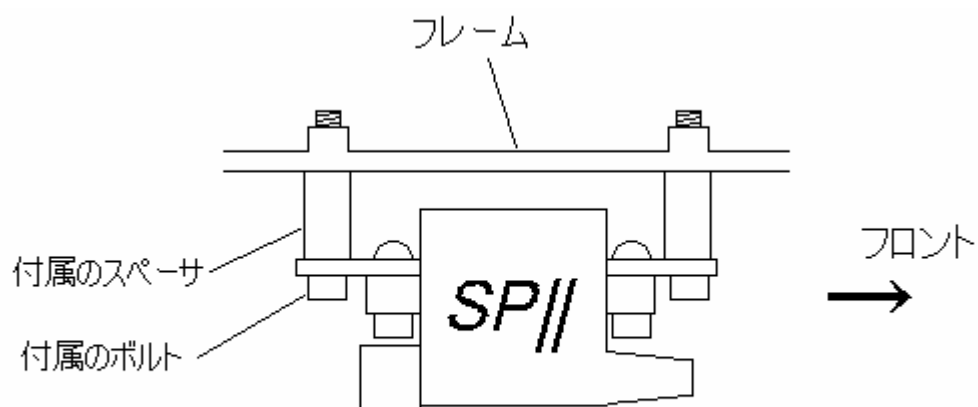
SP II コイル取付図
