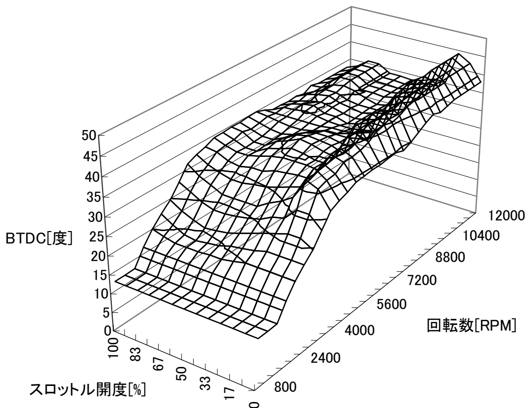
SP II 点火マップ(0マップ) K.ZEPHYR750-2
