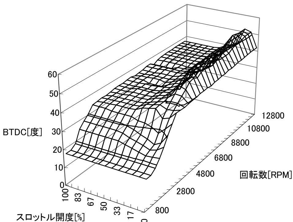
SP II 点火マップ(0マップ) K.ZEPHYR400KAI
