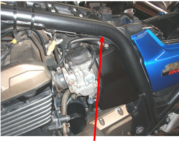
図3、パルシングコイルのコネクタ(2極T型、黒)
