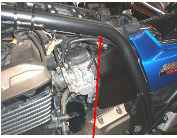
図3、パルスコイルのコネクタ(2極T型、黒)
