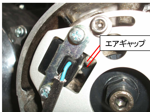
図5、エアギャップを0.4～0.6 mmに 合わせる
