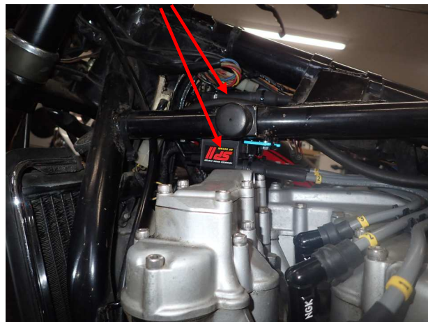
図4 SP II コイルの取付
