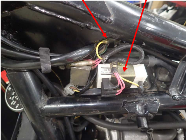
図3 電源(黄ギボシ) レジスタ
