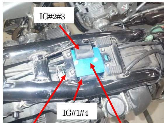
図4、SPⅡコイルの取り付け
