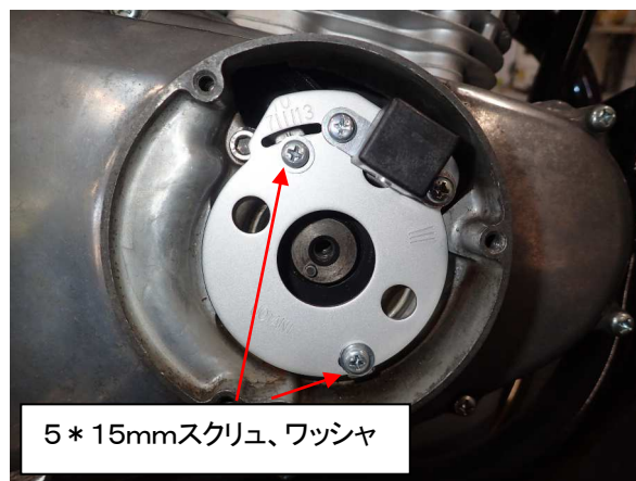
図2、SP II タイミングプレート(ピックアップコイル)の取り付け
