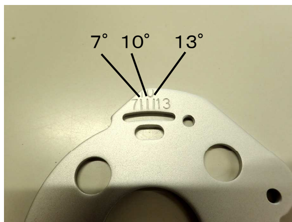
図3、取付スクリュの中心が10° のマークに一致するように装着する
