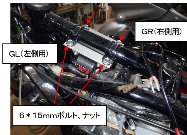
図6、SP II コイルの装着
