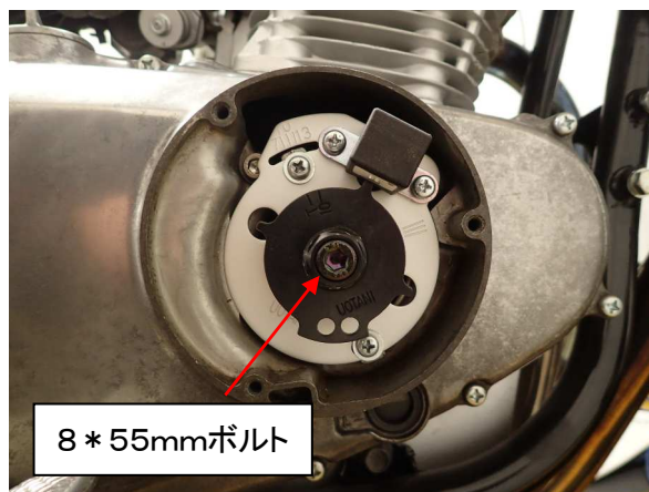
図4、タイミンゴロータの取付
