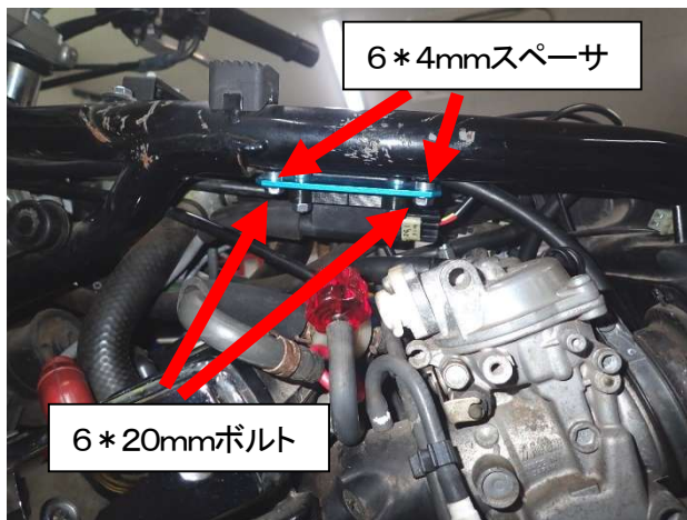
図3、SP2 コイル(1・4)白コネクタ の取り付け
