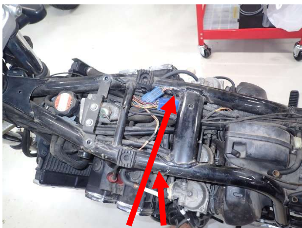
図1、ノーマルコイルの取り外し
