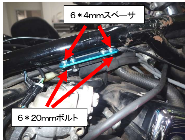
図4、SP2 コイル(2・3)黒コネクタ の取り付け
