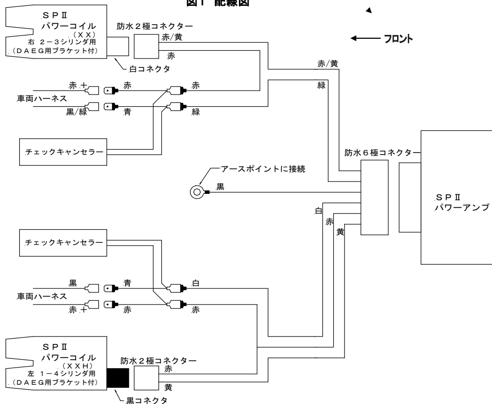
図1 配線図
