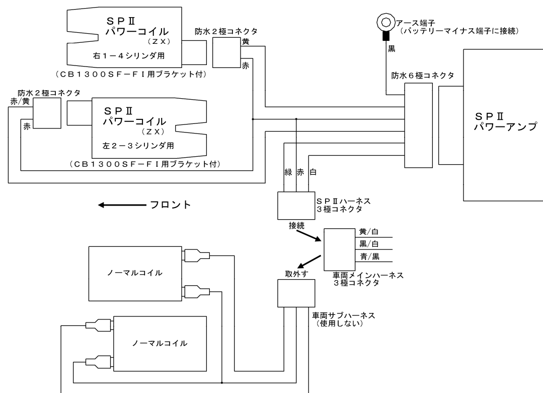
図2 配線図
