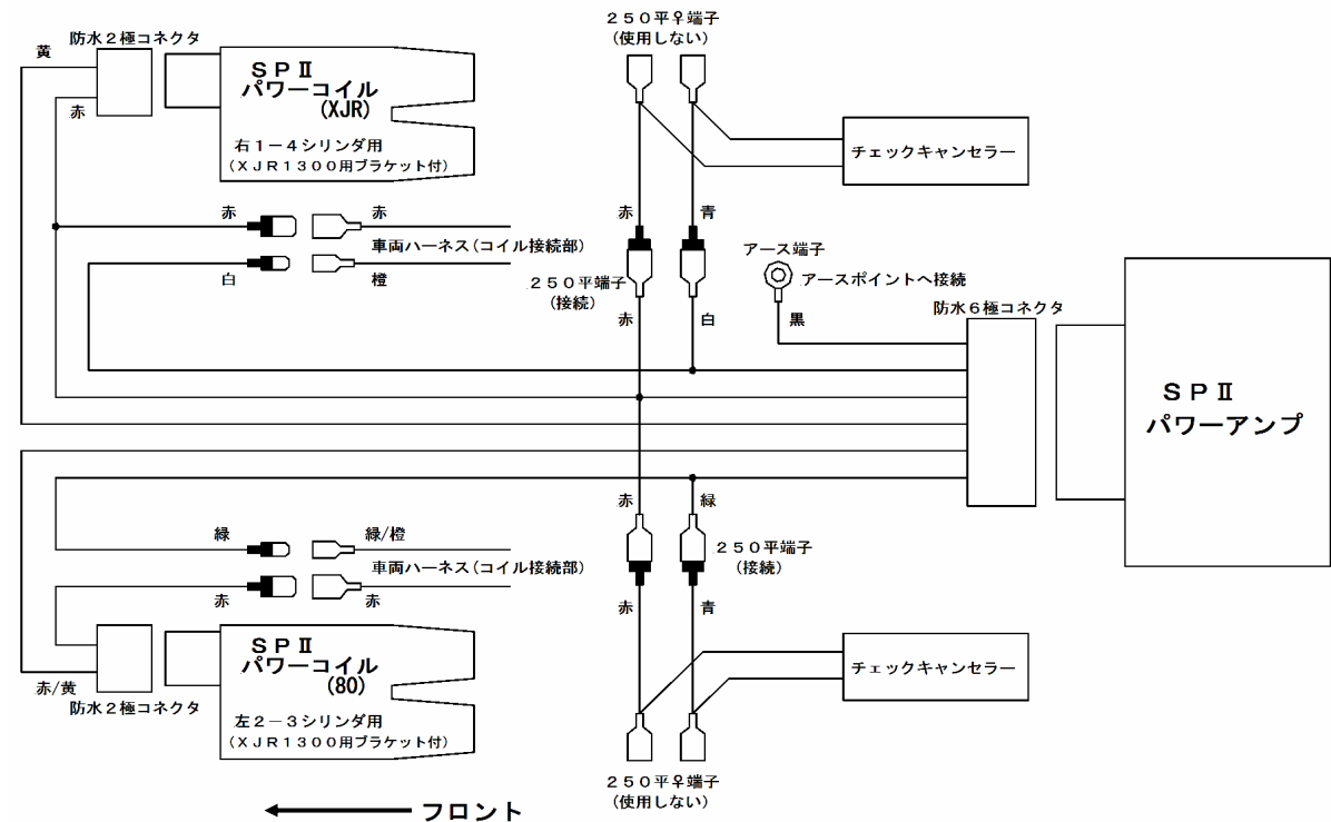
図2 配線図
