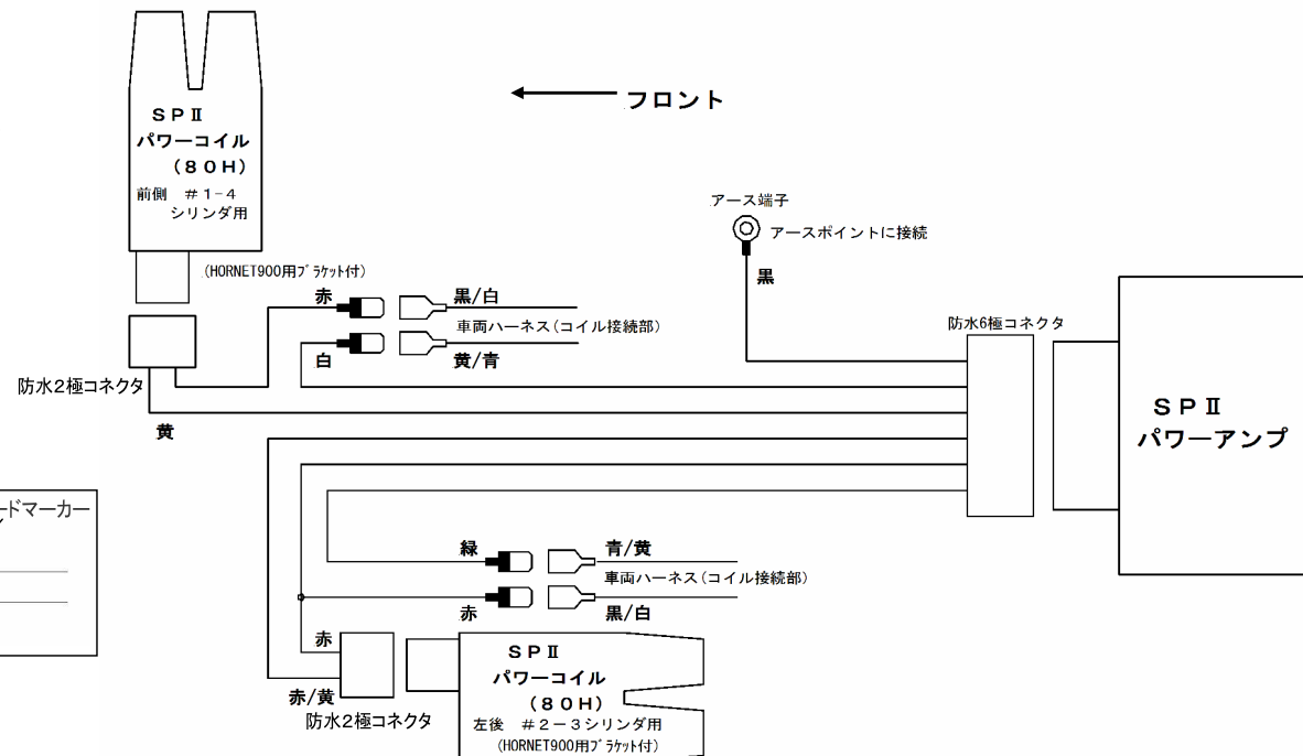
図2 配線図
