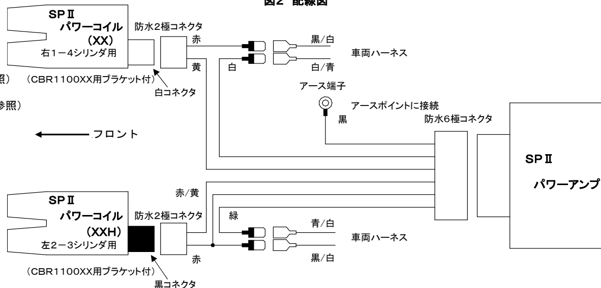
図2 配線図
